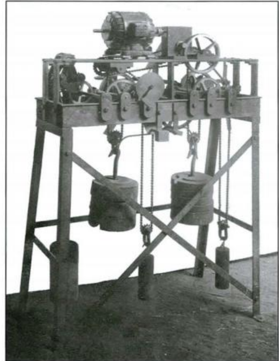
Het "oude" mechanisme voor de bediening van het torenuurwerk.
