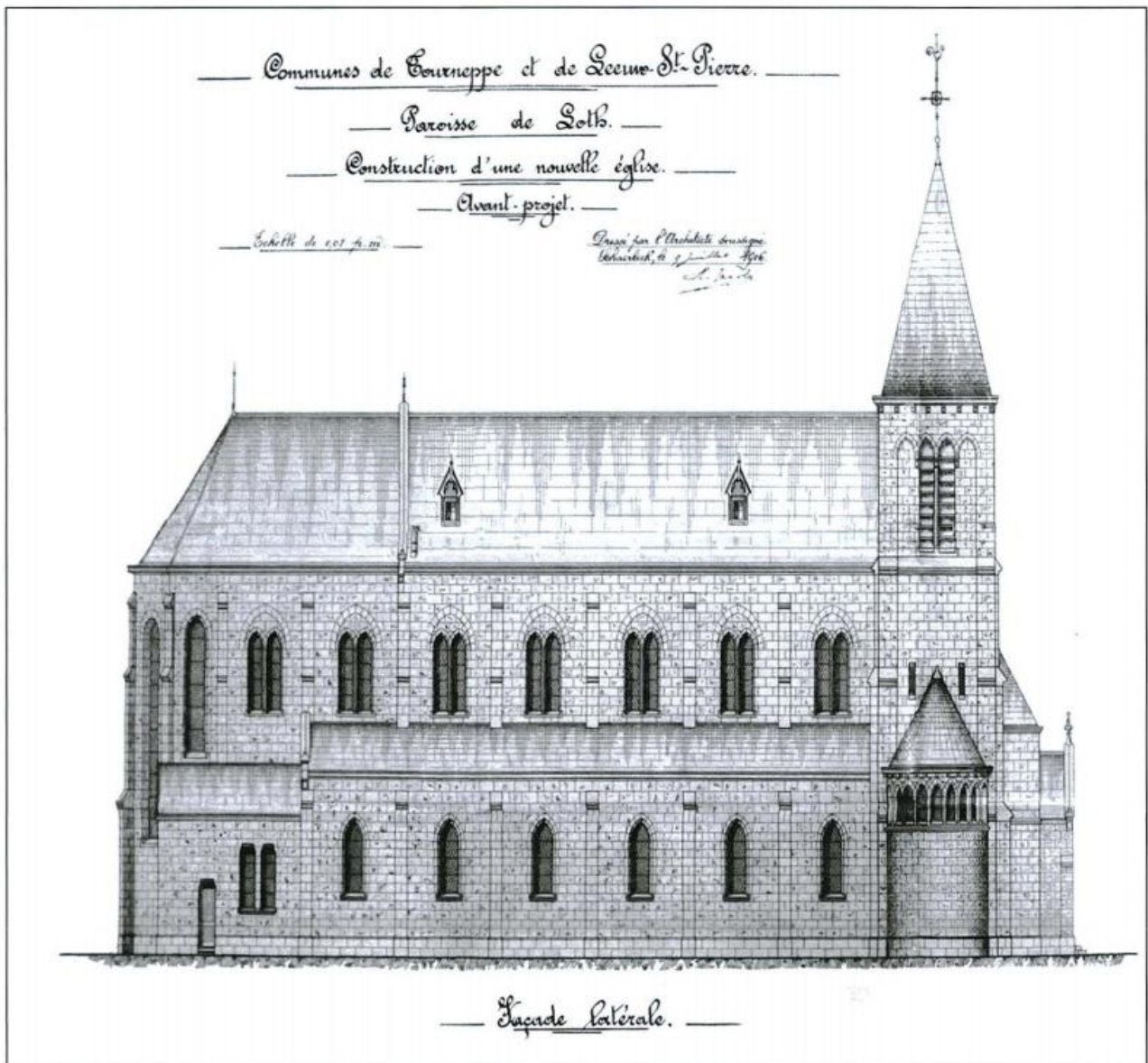
Het ontwerp voor een nieuwe kerk in Lot van architect H. Jacobs, de ontwerper van de nieuwe pastorie.
