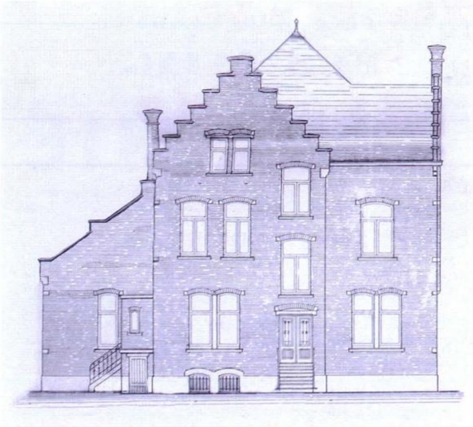
Blauwdruk van een achtergevel van het plan van de pastorie - Henri Jacobs.
